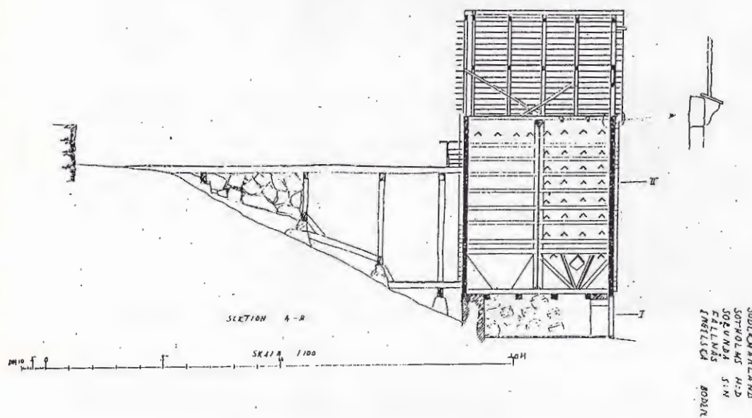
Ritning av "Engelska boden" upprättad i samband med Nordiska museets uppmätning av Fällnäs. Anckarsvärds silo (kornskruv) efter engelskt mönster från omkr. 1820.
